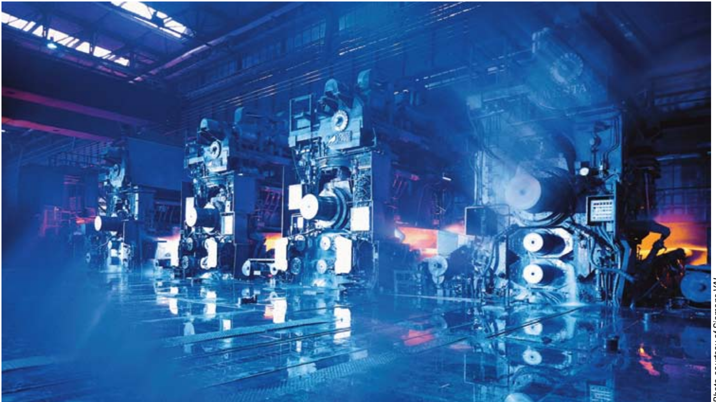
Siemens VAI hot strip mill, Linz, Austria.
